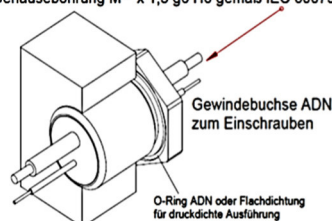
Gehäusebohrung M** x 1,5 g6 H6 gemäß IEC 60079-0
