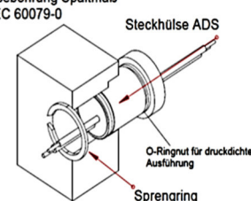
Gehäusebohrung Spaltmaß nach IEC 60079-0
